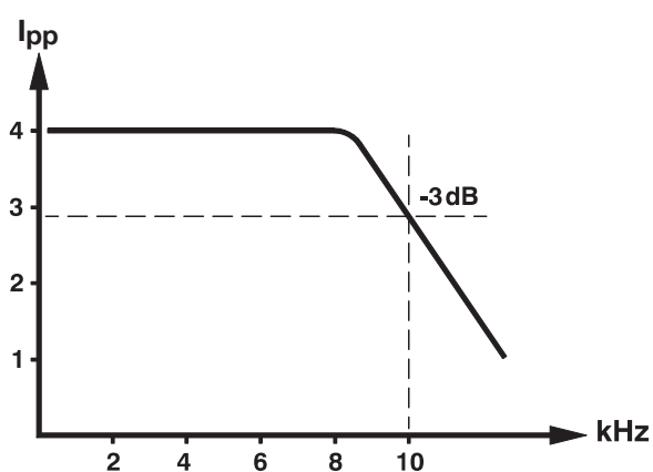
Kleinsignalbandbreite (CC) bei TOE 7621-20
