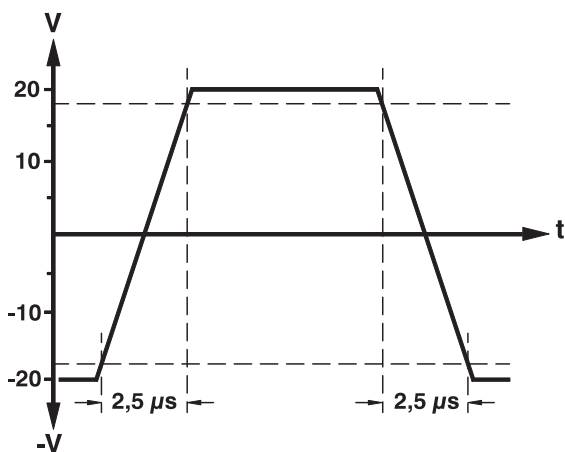
Anstiegs-/Abfallzeit (CV) bei TOE 7621-20
