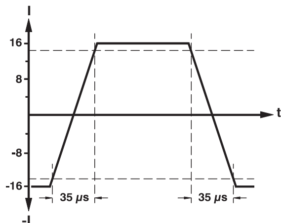
Anstiegs-/Abfallzeit (CC) bei TOE 7621-20
