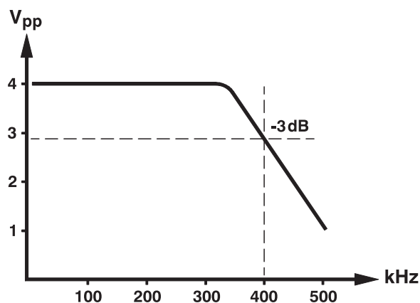
Kleinsignalbandbreite (CV) bei TOE 7621-20
